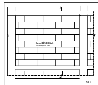
DELTA Block Wall Details N.T.S.
