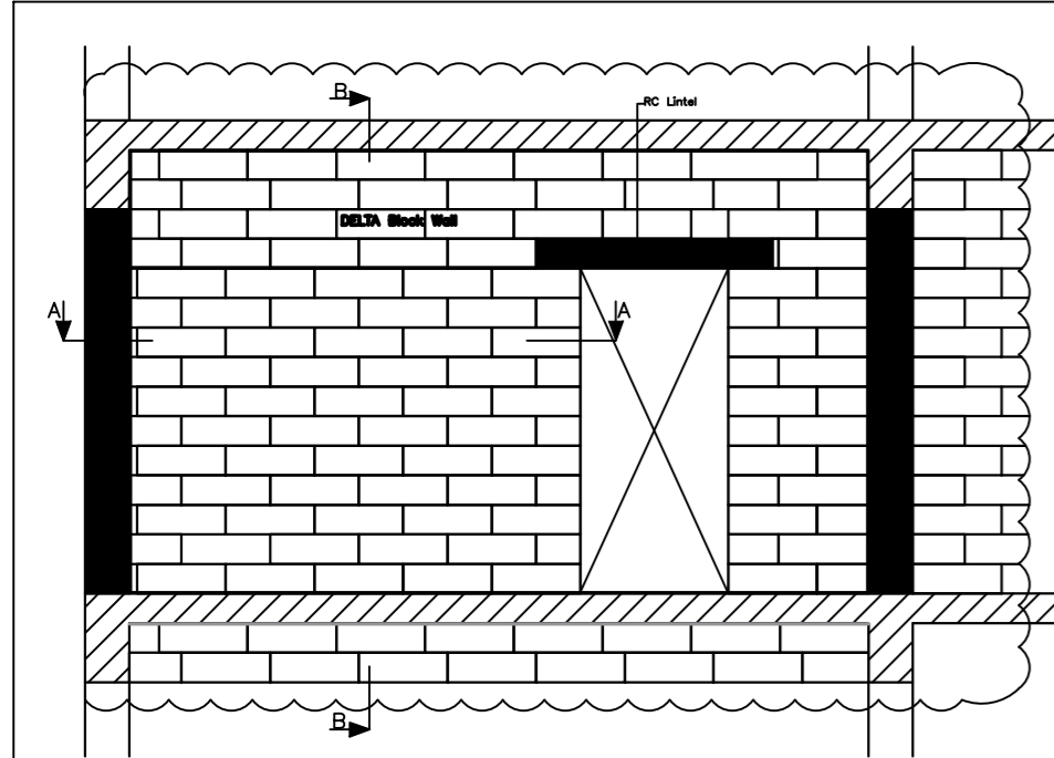
DELTA Block Wall Details N.T.S.
